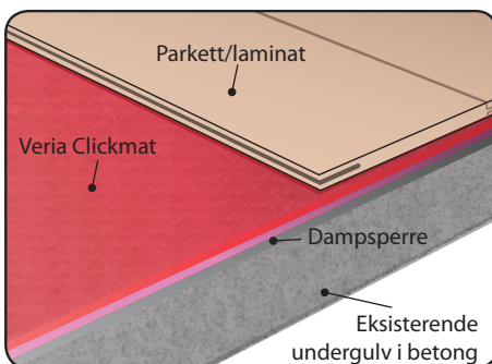
Veria Clickmat på betonggulvkonstruksjon
