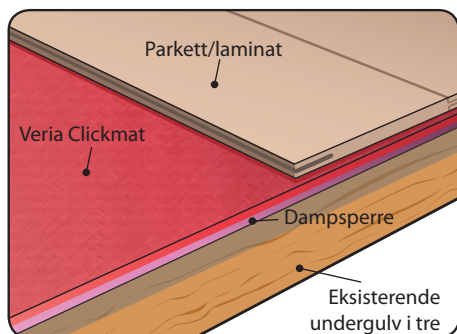
Veria Clickmat på tregulvkonstruksjon
