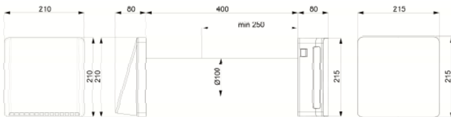
TEMPERO ECO 100
