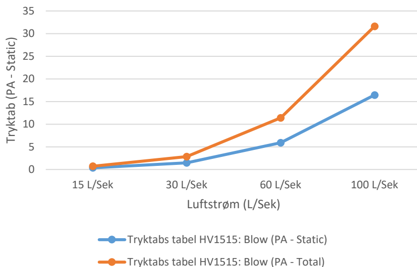
Tryktabs HV15x15 med rundt ISO-rør (Luft ud)
