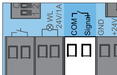
Fig. 5. Tilslutningsklemme til en 2-leder-fotocelle
