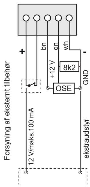
Fig. tilslutningsplan løbevogn
