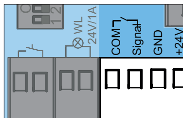
Fig. 6. Tilslutningsklemme til en 4-leder-fotocelle
