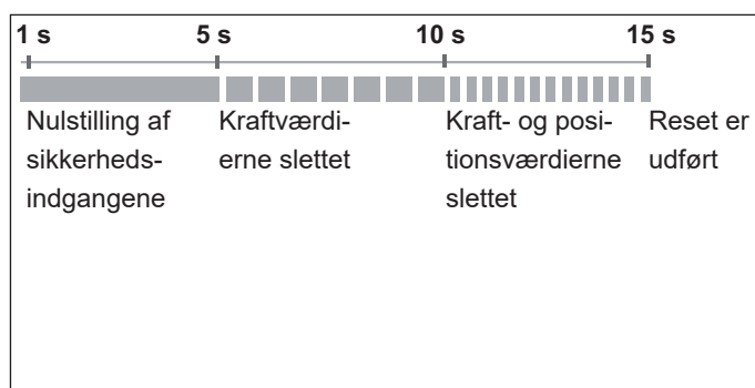
Fig. Oversigt over løbevoignens status-LED's rækkefølge ved tryk på den grønne reset-knap
