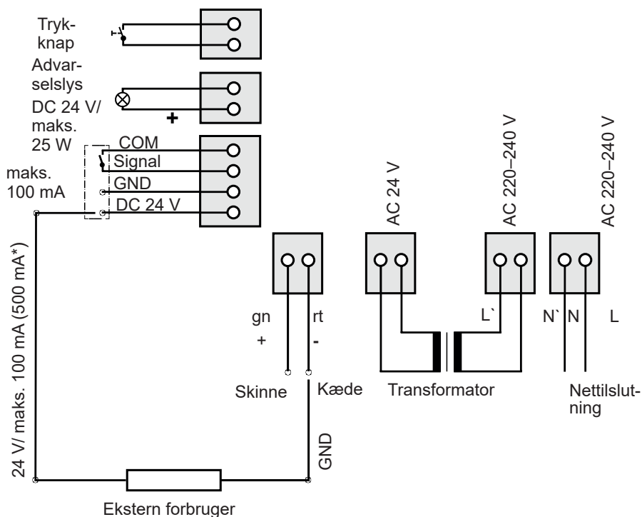
Fig. Tilslutningsplan Loftstyring
