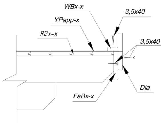
Установка реек для кровельного материала и торцевых досок:
